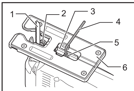
► 1. Hoja de sierra 2. Rodillo 3. Retenedor 4. Llave hexagonal 5. Tornillo 6. Base
