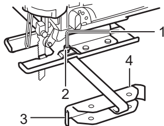
1. Clé hexagonale 2. Boulon 3. Garde parallèle (règle de guidage) 4. Orientation du guide
