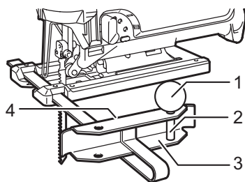
1. Bouton fileté 2. Broche 3. Garde parallèle (règle de guidage) 4. Guide de garde
