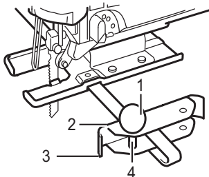
1. Bouton fileté 2. Orientation du guide 3. Garde parallèle (règle de guidage) 4. Broche
