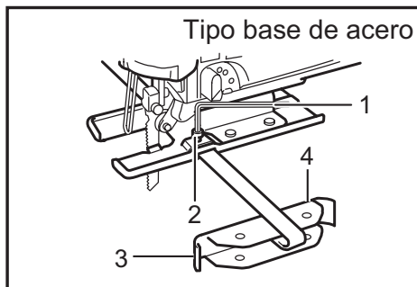
1. Llave hexagonal 2. Tornillo 3. Guía lateral de corte (regla de guía) 4. Revestimiento de guía
