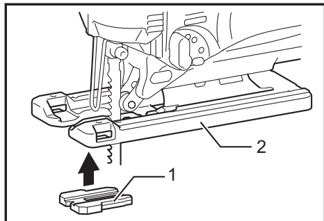
► 1. Dispositivo antiastillado 2. Base de aluminio
